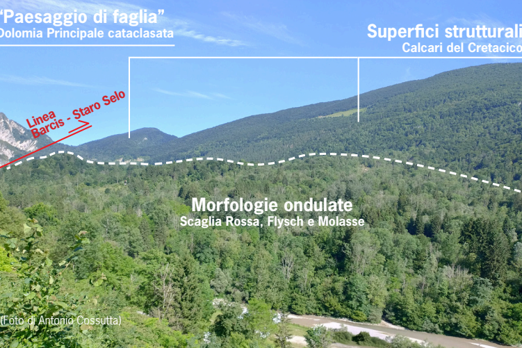
Superfici strutturali, morfologie ondulate e "paesaggio di faglia" Structural surfaces, undulating forms and "fault terrain"
